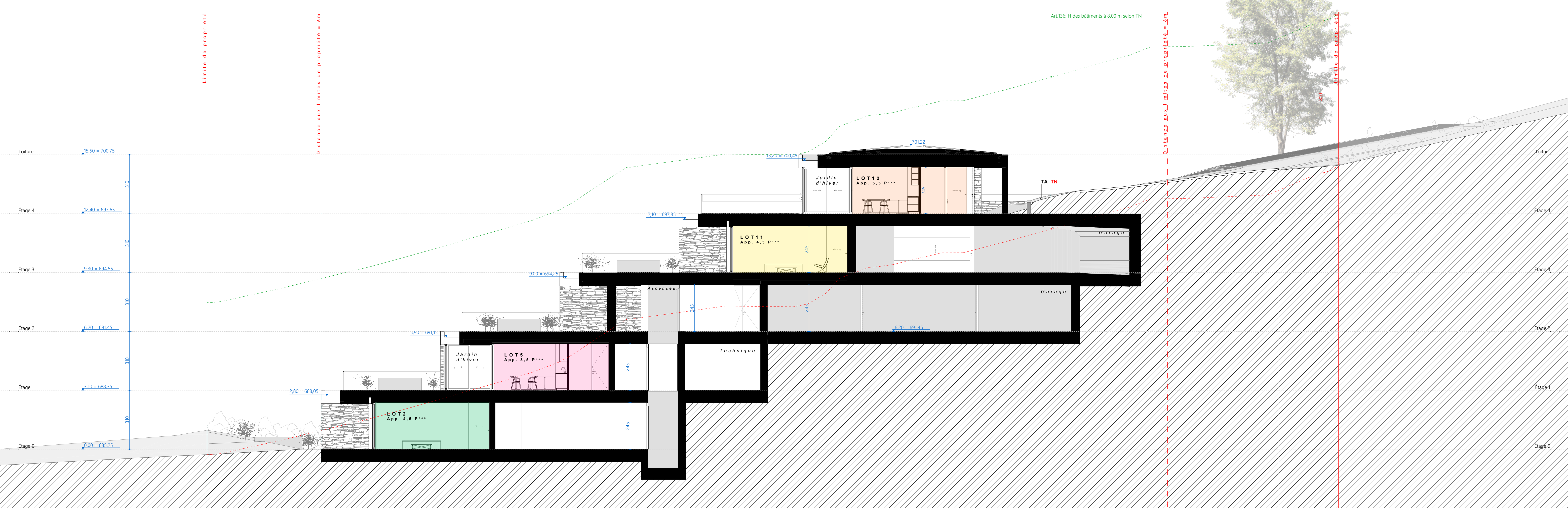
Coupe 02
