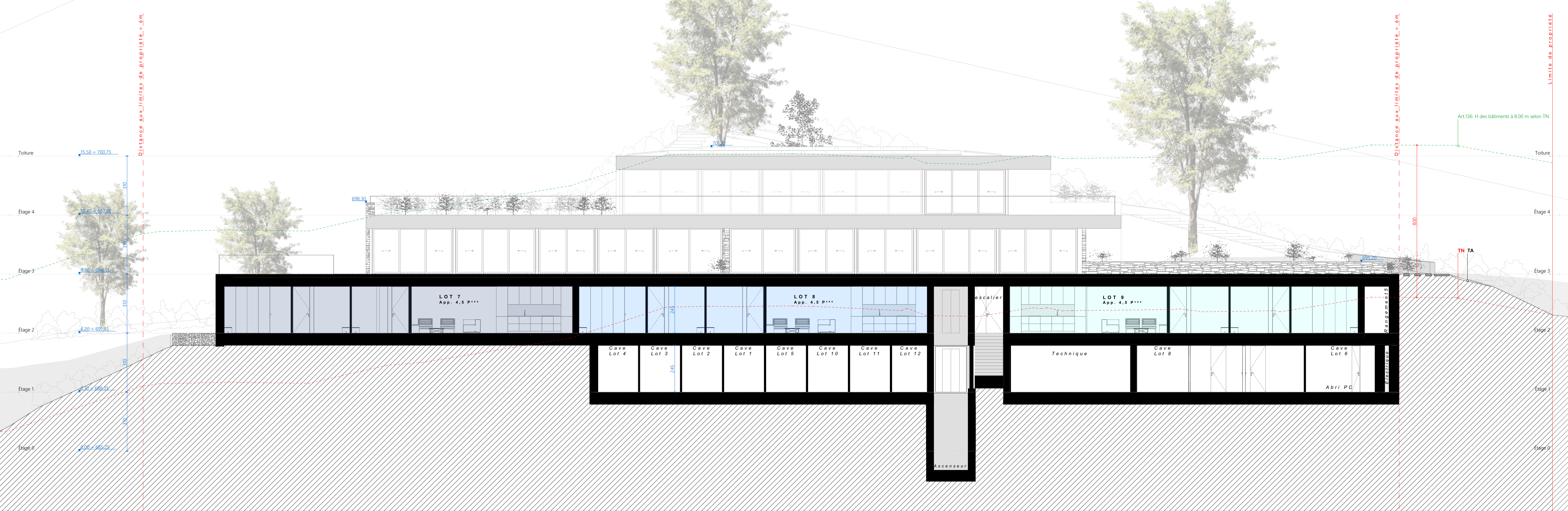
Coupe 04
